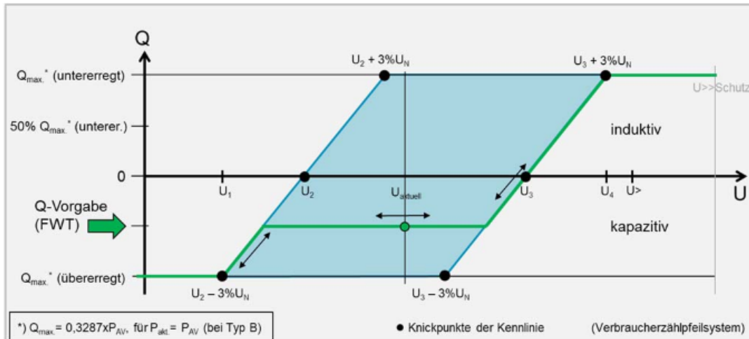
Bild 2.6: Q(U) -Verhalten für eine EZA vom Typ A bei Q\text{-Soll} = 0,5 \times 0,3287 \times P_{AV} kapazitiv (übererregt)
