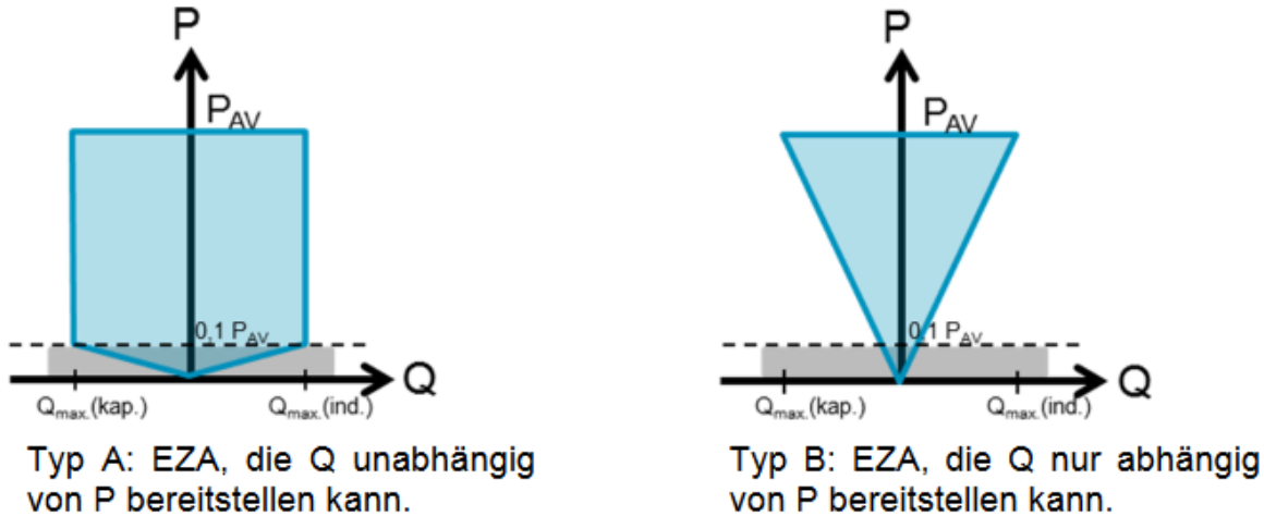
Bild 2.2: Unterscheidung des Blindleistungsvermögens von EZA nach Typ A und Typ B
