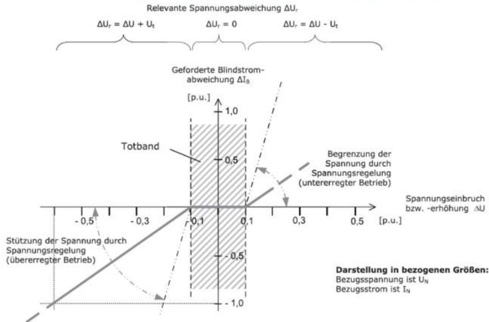
Bild 3.6: Prinzip der Spannungsstützung bei Netzfehlern bei Windenergie-Erzeugungseinheiten
