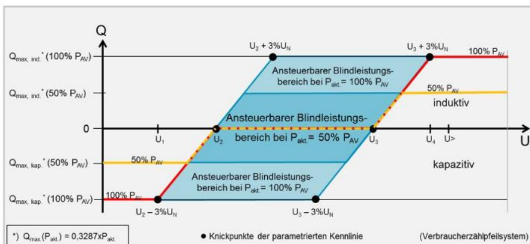
Bild 2.5: EZA vom Typ B: Q(U)-Verhalten (orange) bei P_{akt.}=50\%P_{AV} und Q\text{-Soll}=0 sowie der ansteuerbare Blindleistungsbereich (dunkelblau) für Q\text{-Soll}\neq 0 ; Q(U)-Verhalten (rot) bei P_{akt.}=100\%P_{AV} und Q\text{-Soll}=0 sowie der ansteuerbarer Blindleistungsbereich (hell- und dunkelblau) bei Q\text{-Soll}\neq 0
