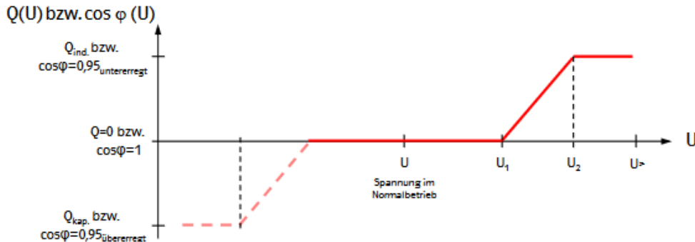
Bild 9.1: Qualitative Darstellung des spannungsabhängigen Blindleistungsverhaltens von Erzeugungsanlagen
