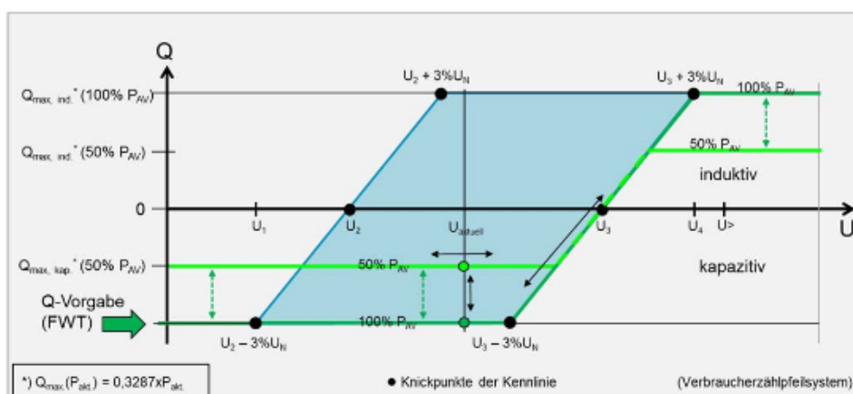
Bild 2.8: Q(U)-Verhalten für eine EZA vom Typ B bei Q-Vorgabe von 0,3287 \times P_{AV} kapazitiv (übererregt) und P_{akt} = 50\% P_{AV} (hellgrüne Linie) sowie P_{akt} = 100\% P_{AV} (dunkelgrüne Linie)
