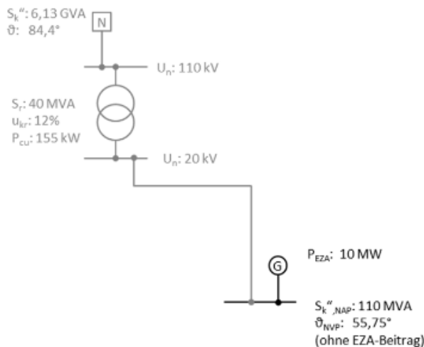
Bild 8.1: Testsystem zur Bewertung des Regelungsverhaltens
