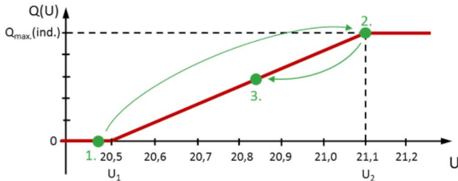
Bild 8.2: Q(U) -Kennlinie für Testsystem
